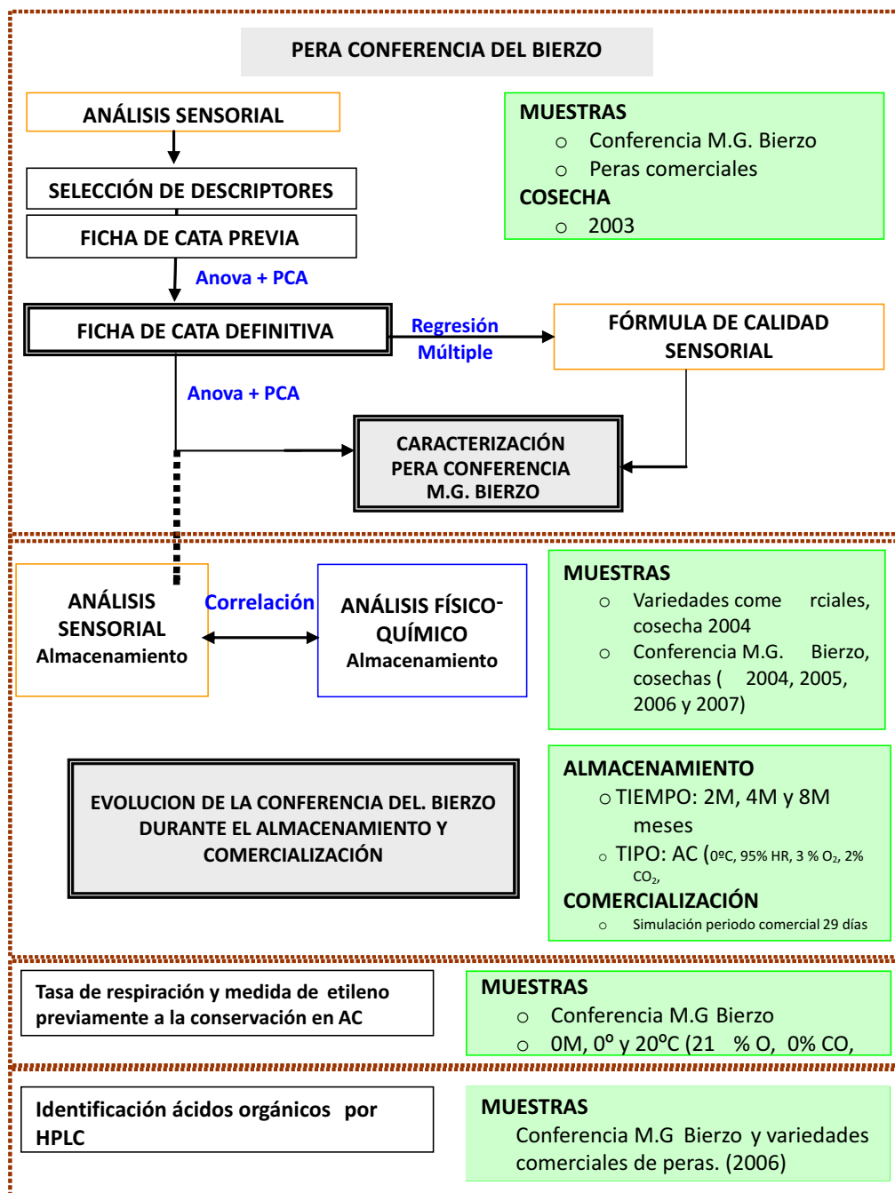
Fig.3.4. Esquema general del proceso experimental llevado a cabo para la Conferencia M.G. del Bierzo (León).
