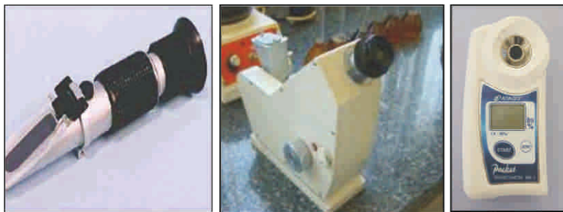
Fig.2.32. Diferentes equipos para la medición de grados brix.
